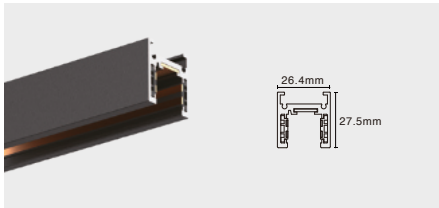
TLS-ECO-MS2X0 (X:1/ 2 / 3M)
